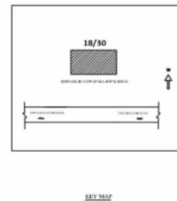
SKY MAP
